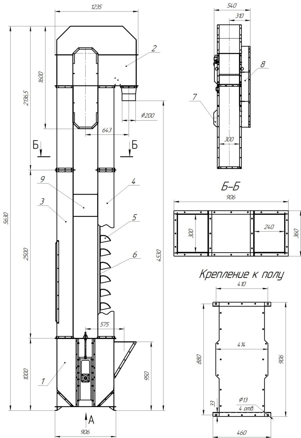
Нория ковшовая габаритные размеры
